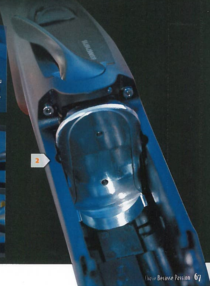
1. 2. Deux plans différents du bloc de verrouillage basculant et des petits verrous placés de part et d'autre du bloc
